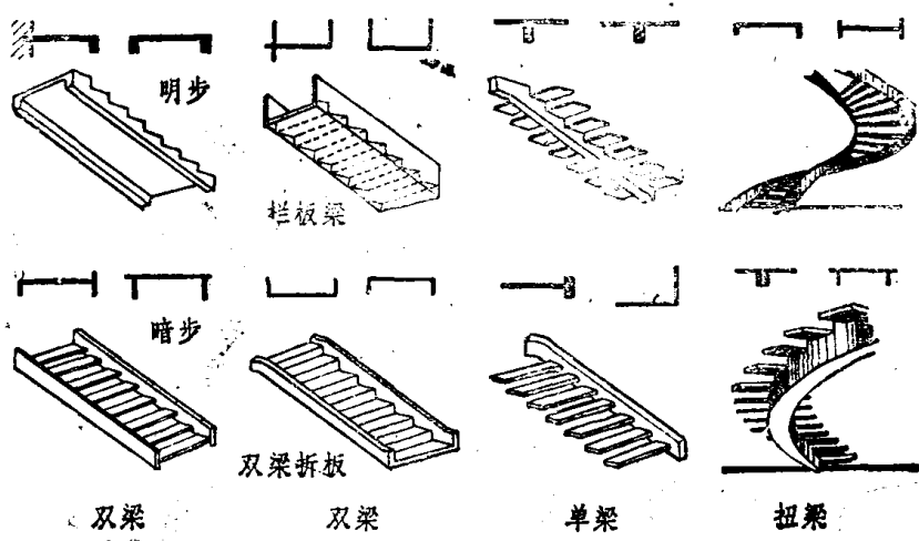
图 1-12 梁式楼梯跑的形式
