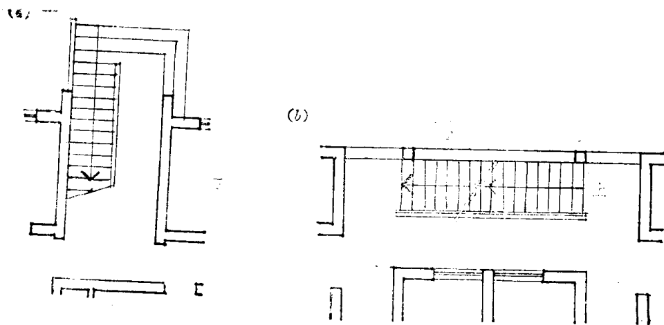
图 1-2 直上楼梯
