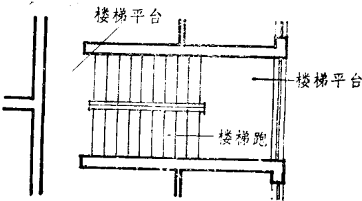
图 1-9 楼梯的组成
