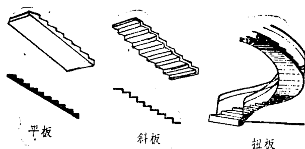
图 1-11 各种板式楼梯跑
