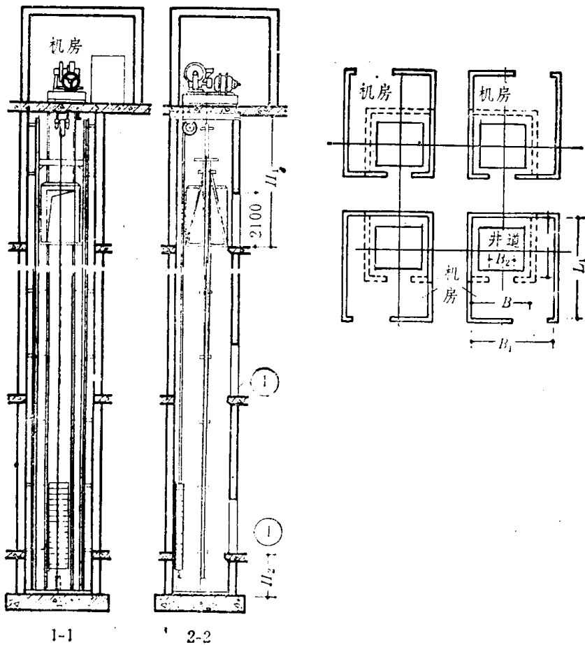
图 1-8 电梯井道和机房平面图
