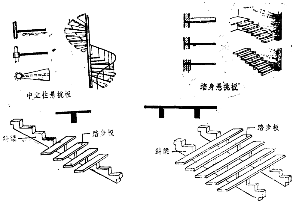
图 1-13 悬臂板楼梯跑的各种形式
