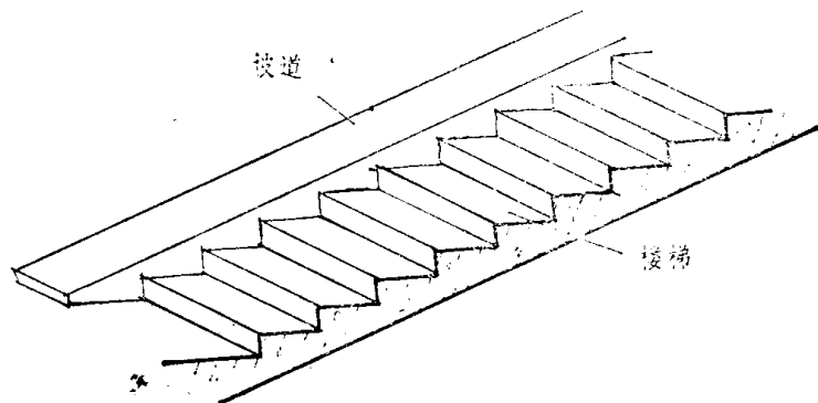
图 1-6 坡道与楼梯的结合
