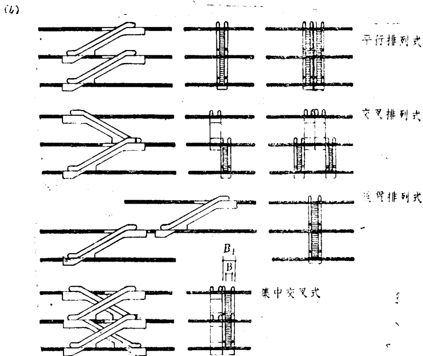
图 1-7 自动楼梯传动示意和布置方式 (a)自动楼梯传动示意；(b)自动楼梯布置方式
