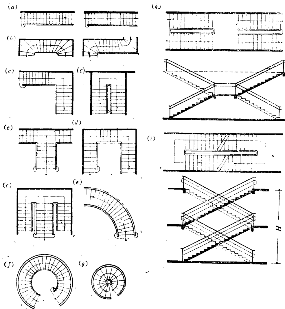
1-1 楼梯的基本形式
