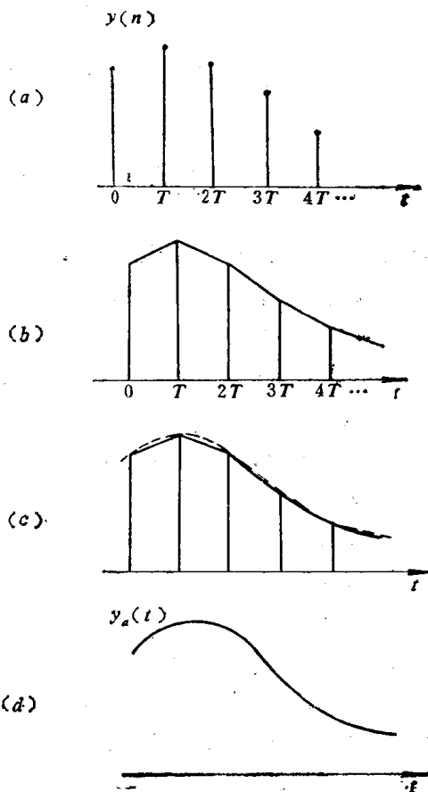
图 1-6 一阶多角形保持法
