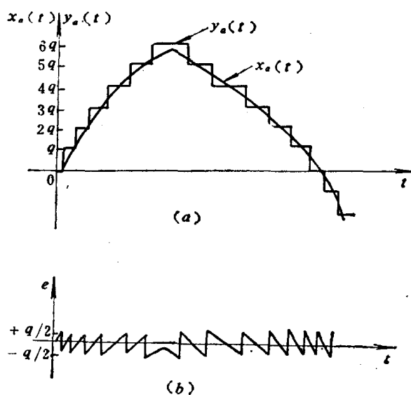
图 1-7 量化及量化误差波形图
