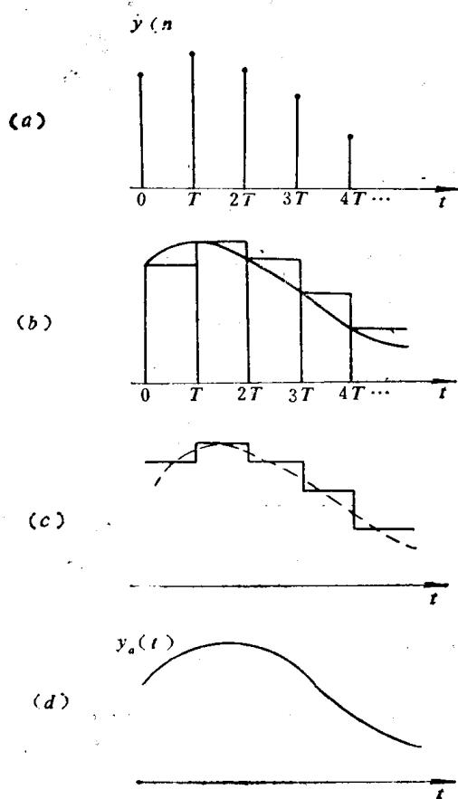
图 1-5 零阶保持法
