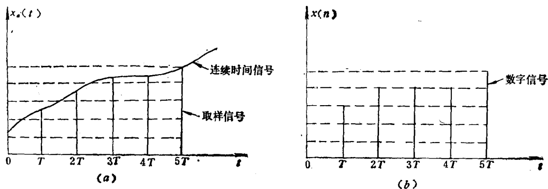
图 1-1 连续时间信号的取样与量化
