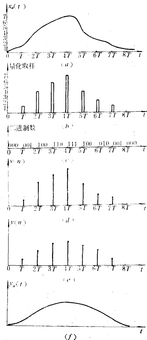
图 1-4 数字信号处理过程波形图
