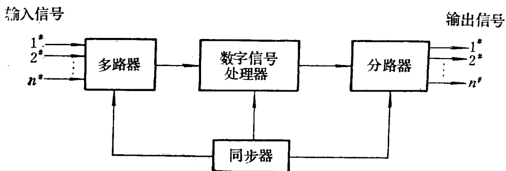
图 1-8 时分复用系统
