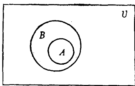
图 1-1 集合的包含关系图
