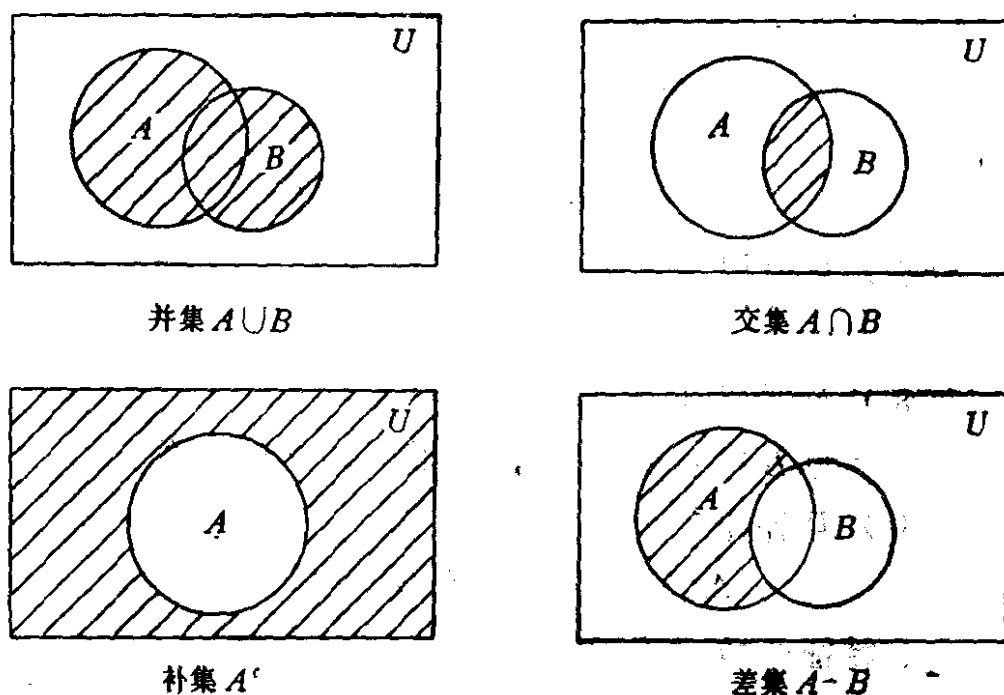
图 1-2 集合运算图
