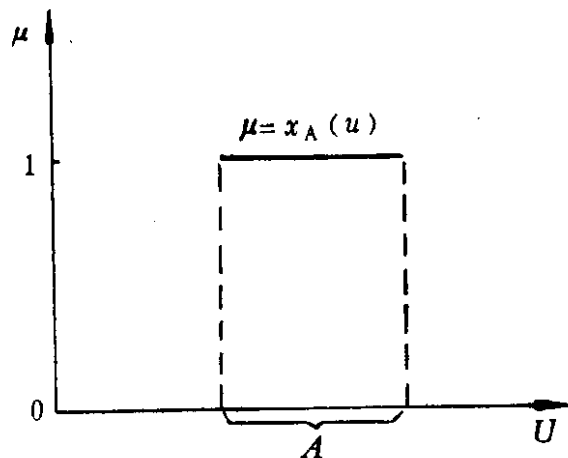
图 1-3 特征函数图
