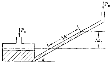
图 1-4 斜管压力计
