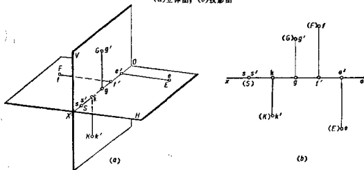
图 1-2 特殊位置点的投影 (a)立体图; (b)投影图
