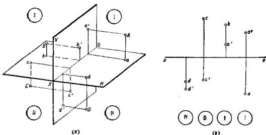
图 1-1 一般位置点的投影 (a)立体图; (b)投影图
