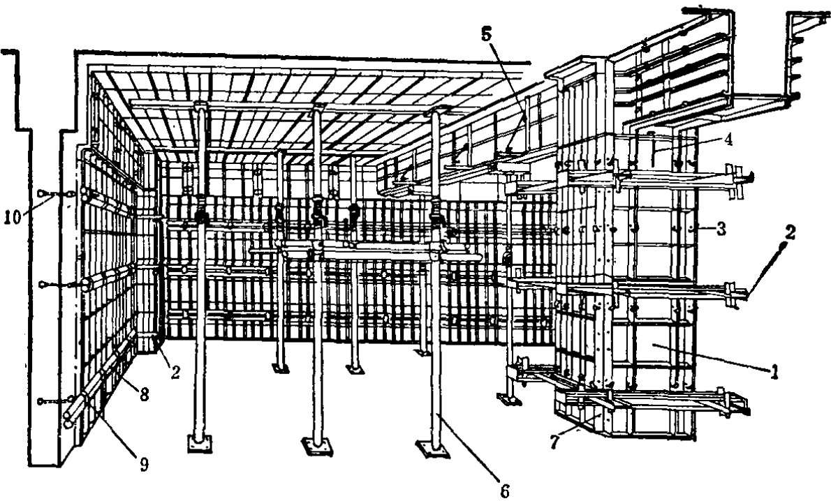
图 1-1 组合钢模板的组成
