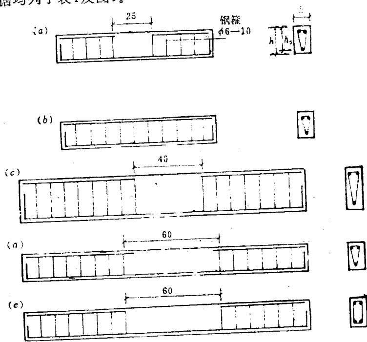
图1 试件配筋率：钢箍全部用 \phi 6 ，间距10cm，压区钢筋 2\phi 8
