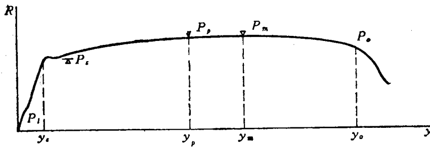
图6 构件的抗力曲线
