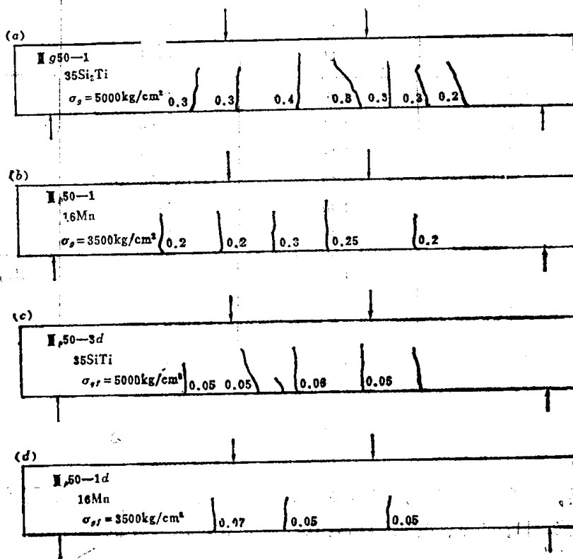
图 8 a、b 静速加载 c、d 爆炸曲线形式加载后 拉区混凝土裂缝情况 (屈服前)
