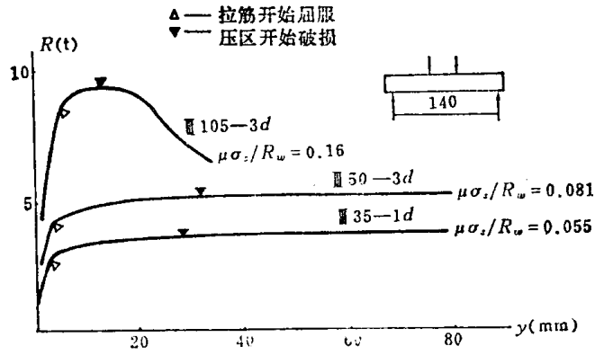
图 11 抗力曲线的典型形状
