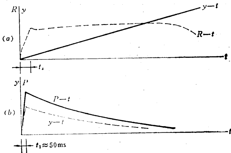
图2 加载方式 P—荷载，y—跨中挠度 (a) 等变形速度加载 (b) 爆炸曲线加载。
