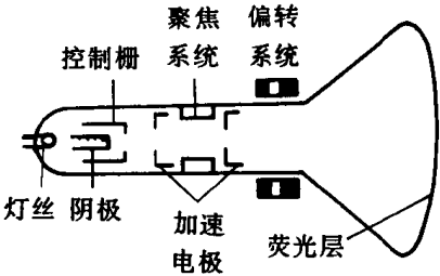
图 1.3.1 阴极射线管示意图
