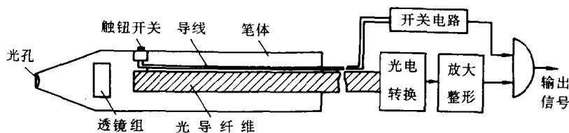
图 1.2.1 光笔结构示意图
