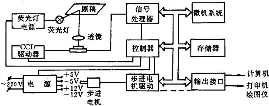
图 1.2.3 扫描仪的模块框图
