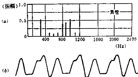
图 1-3 黑管的振动图象和声谱图
