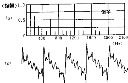
图 1-4 钢琴的振动图象和声谱图
