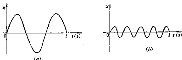
图 1-1 频率为 f 与 3f 的简谐振动
