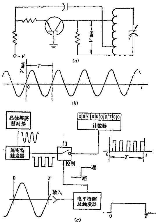
图 2-3 伽利略观测单摆的电子改型
