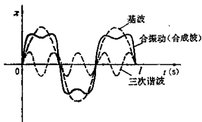
图 1-2 基波与三次谐波的合成
