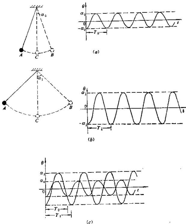
图 2-2 摆的运动
