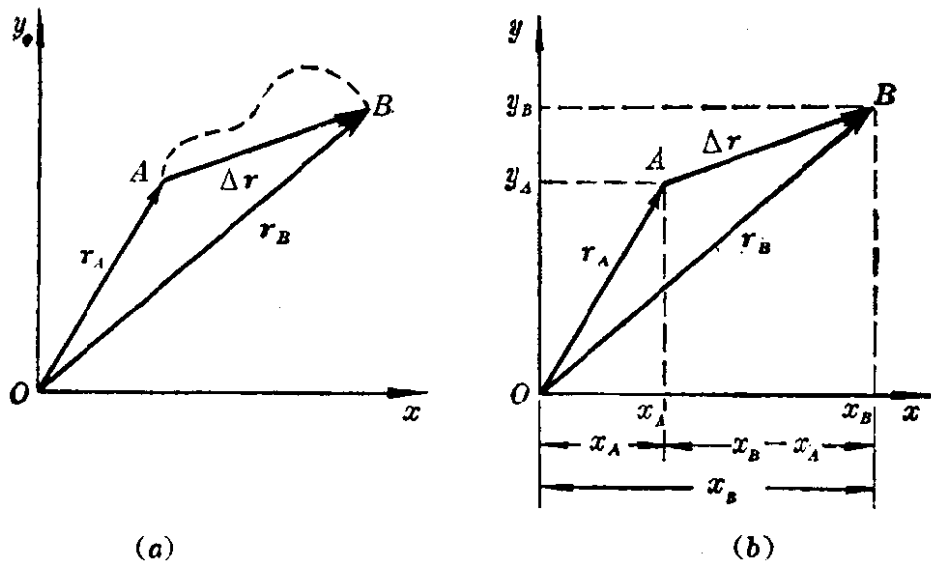
图 1-2 位移矢量
