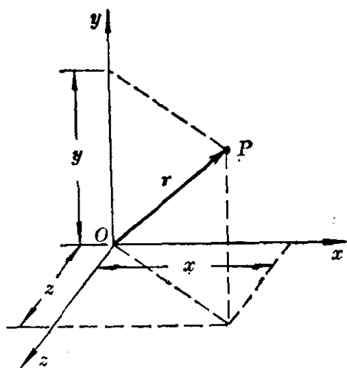
图 1-1 位置矢量
