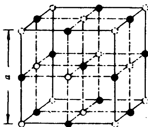
图 1-1 氯化钠结构
