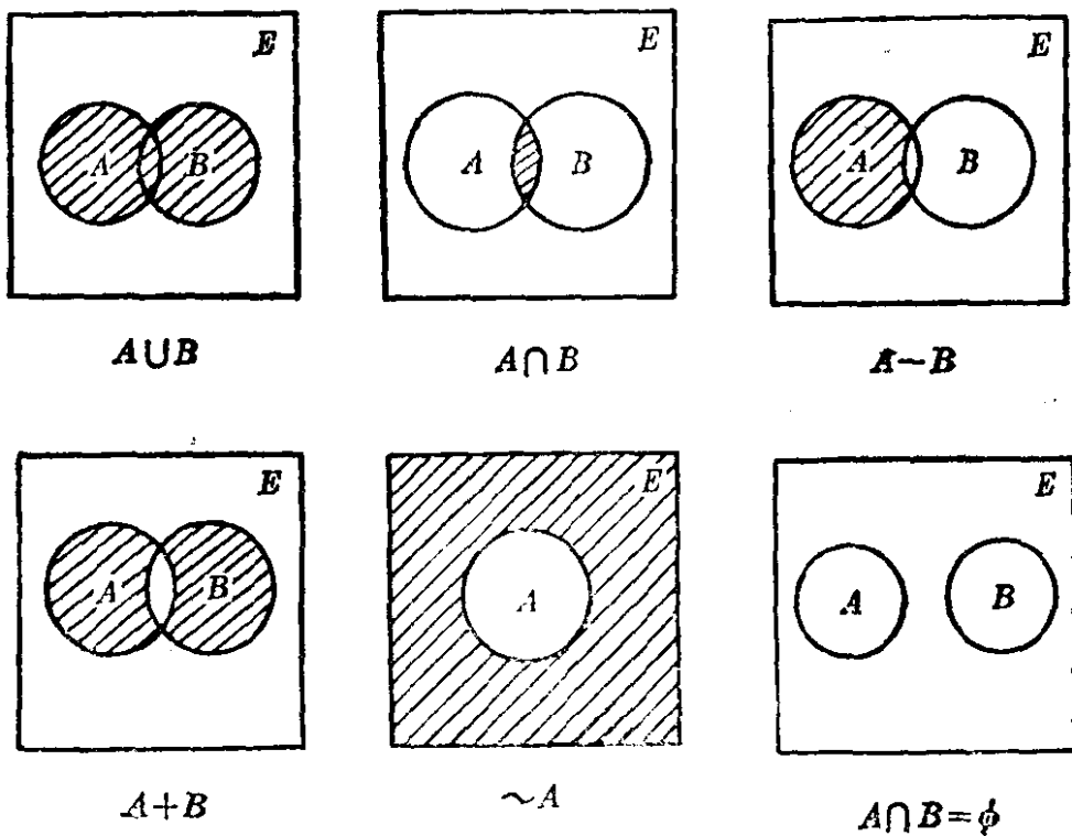
图 2 几种集合运算的文氏图
