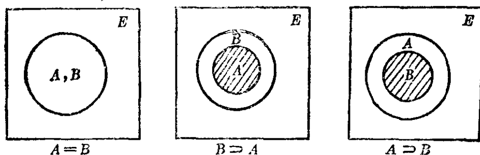
图 1 相等与包含关系之文氏图
