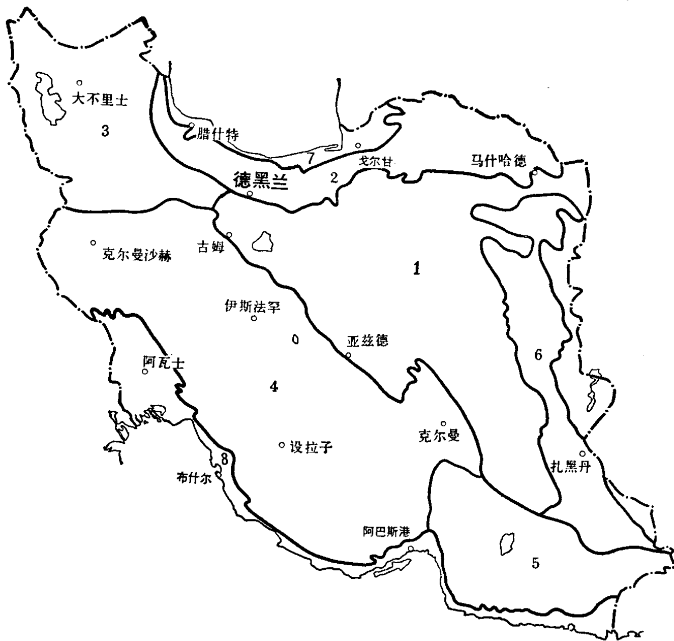
图 5 伊朗地形分区图
