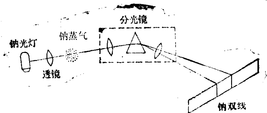
图1—1 原子吸收分析示意图
