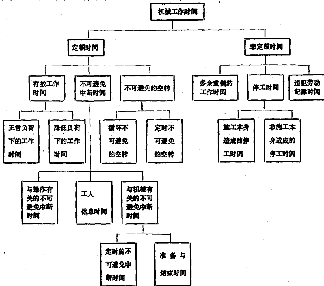
图1-2 机械工作时间分析图
