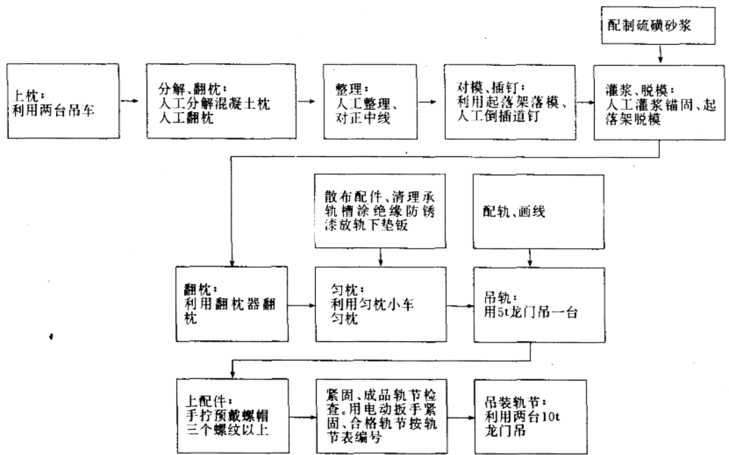
图5 轨节生产工艺流程
