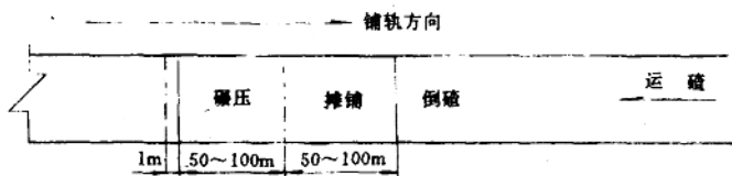
图2 单(双)线单层道床作业示意图
