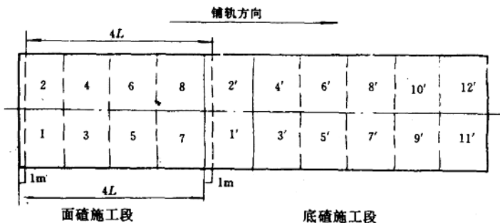
图4 双线双层道床施工区段
