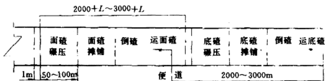
图3 单线双层道床作业示意图
