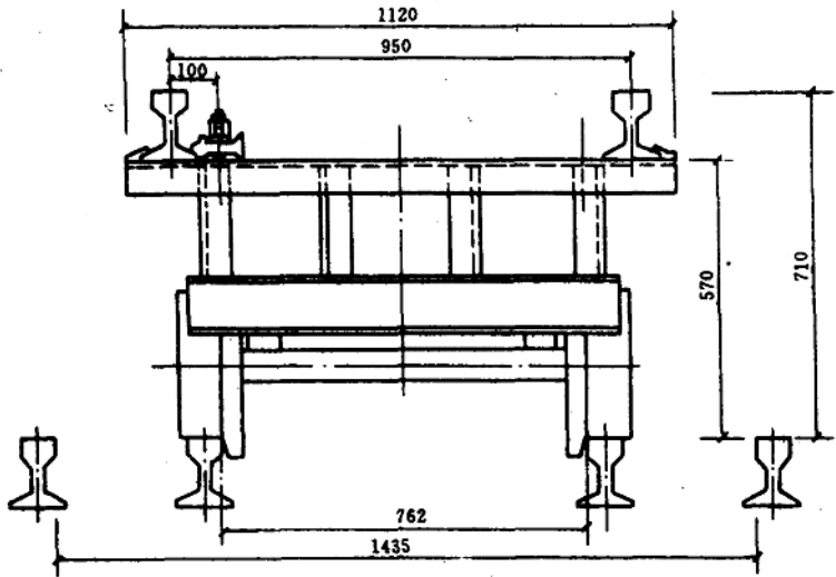
图 2 轨节作业线走行部分布置示意图
