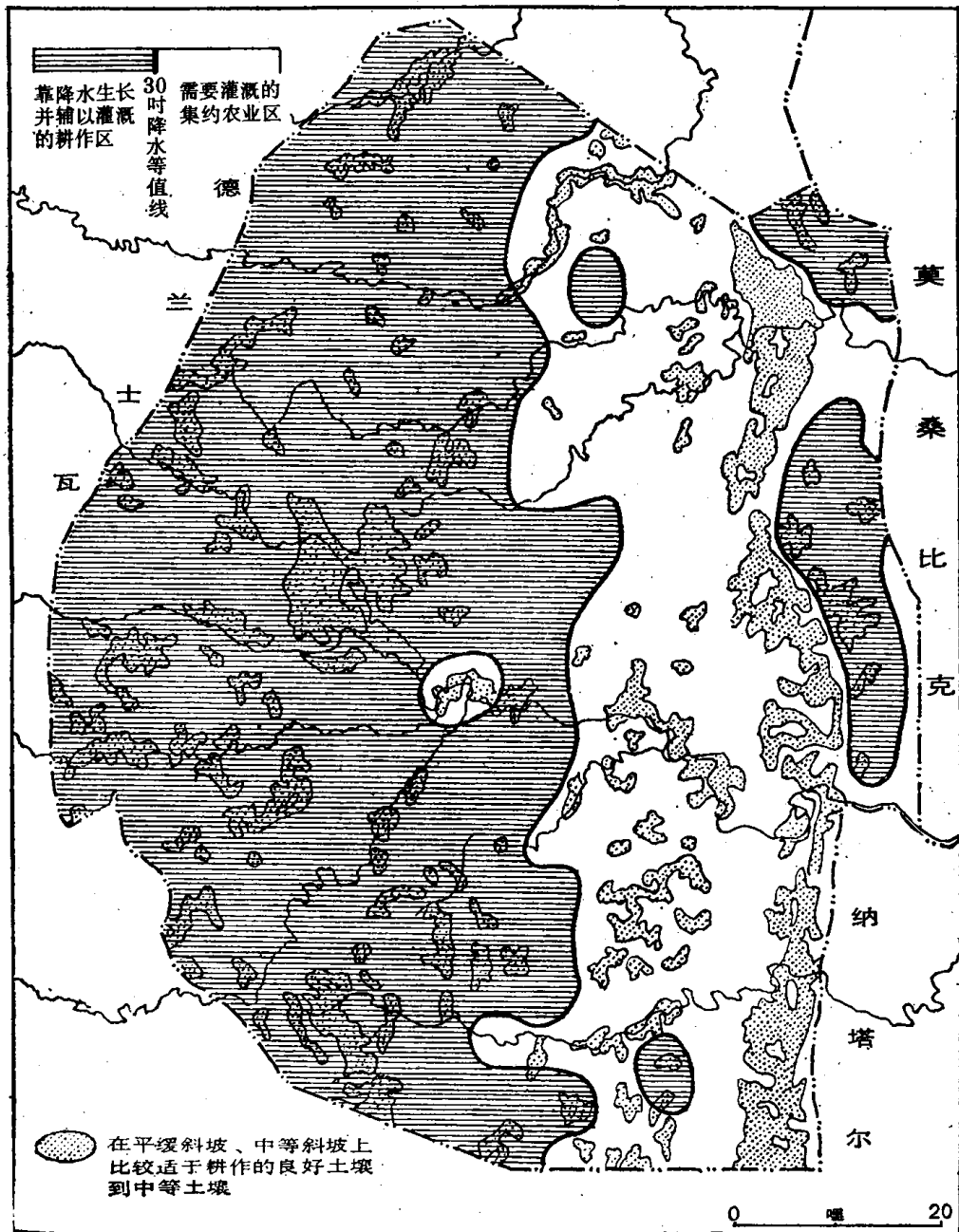
图 2 自然资源基础: 一般土地潜力
