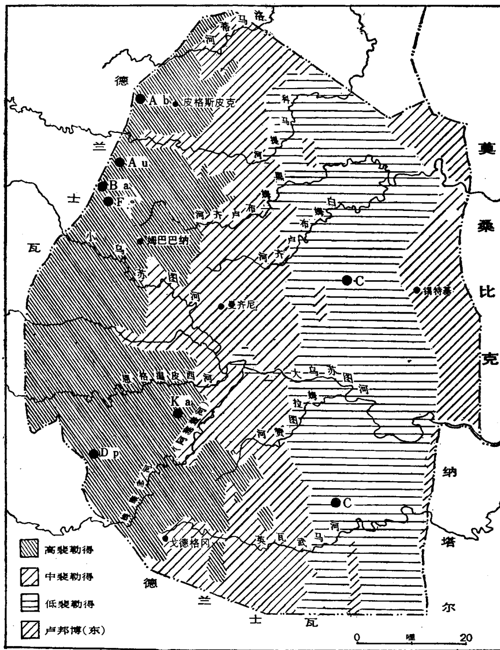
图 1 自然资源基础：自然地理区与矿物
