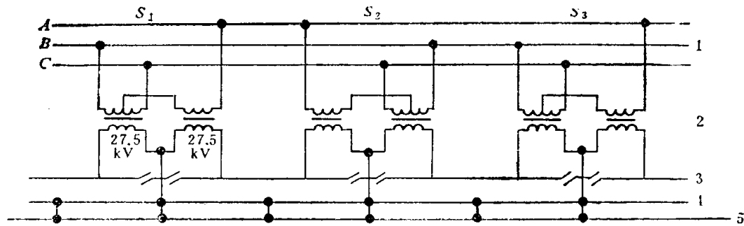
图1-1-8 三相/二相斯科特结线普通牵引变电所原理结线简图
