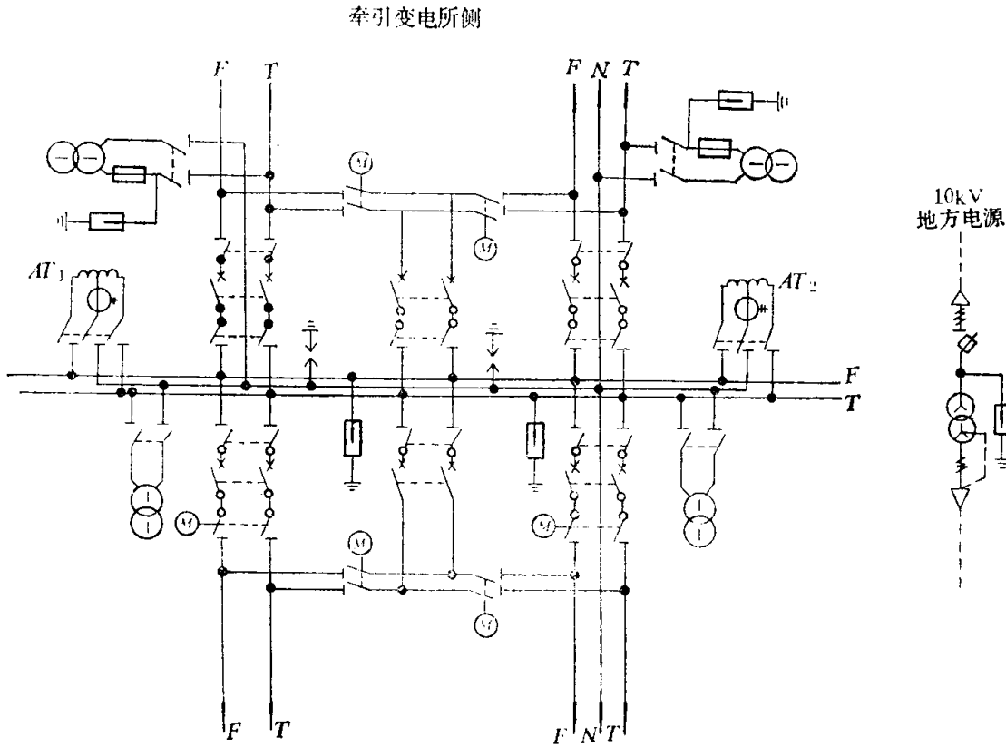
图1-1-9 双线AT开闭所主结线图
