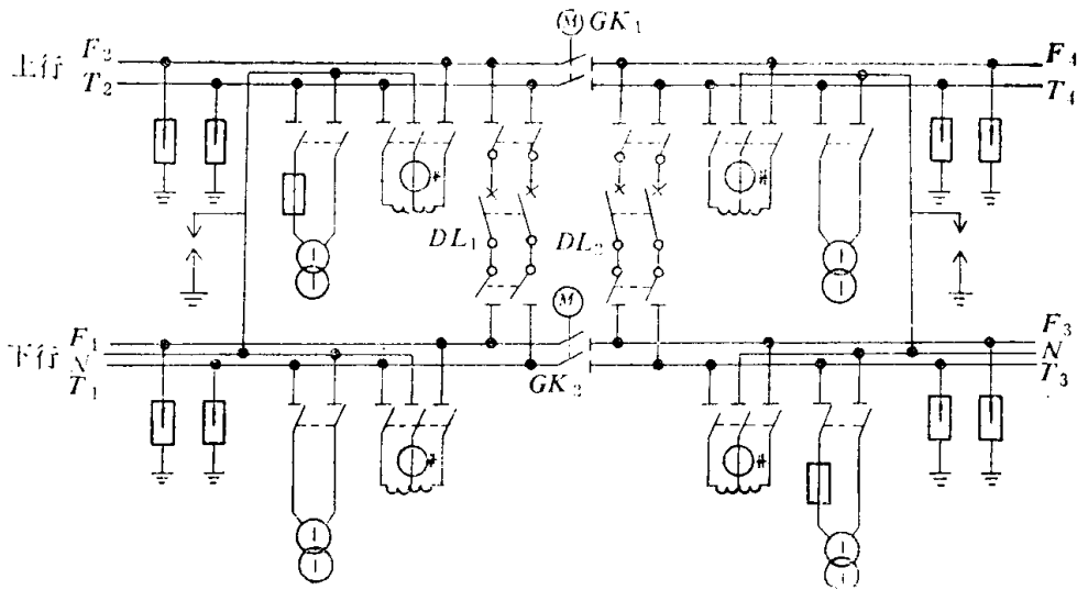
图1-1-10 双线AT分区亭主结线图
