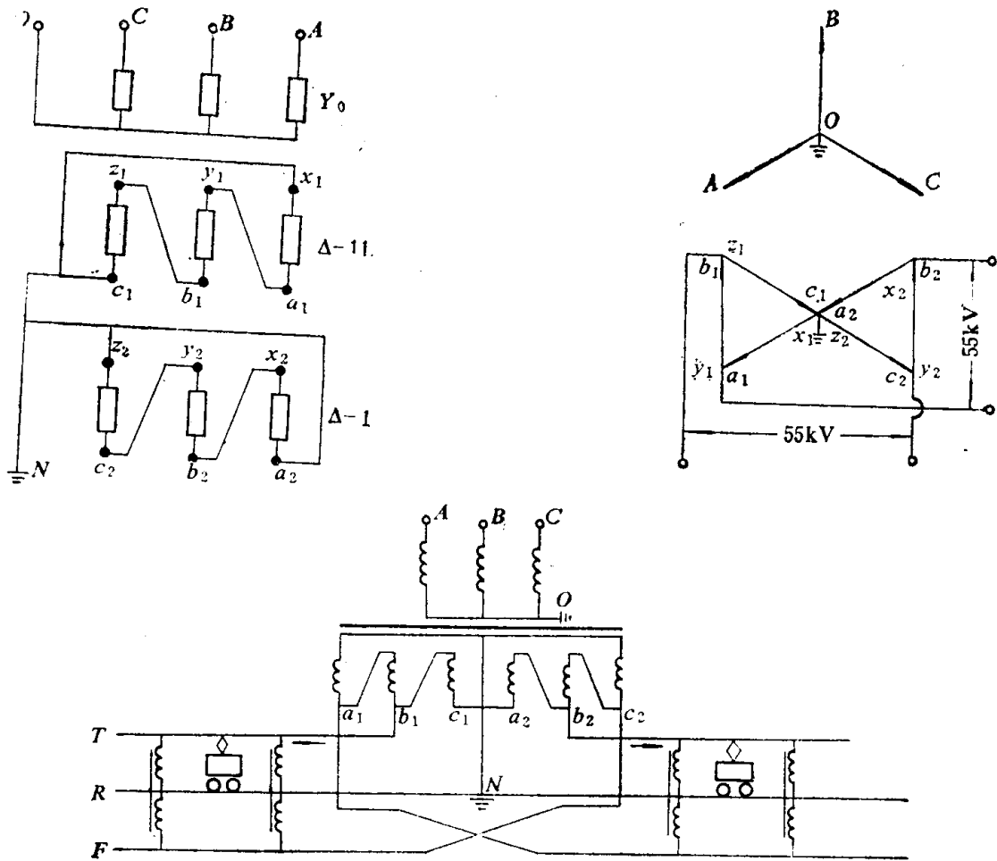
图1-1-4 三相 Y_N 、 d_{11} 、 d_1 十字交叉结线AT牵引变电所原理结线简图
