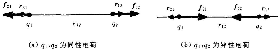
图 1.1 两点电荷 q_1, q_2 间的相互作用力
