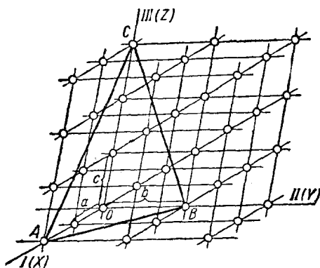
圖 2. ABC 晶面在坐標軸上截整數間距。
