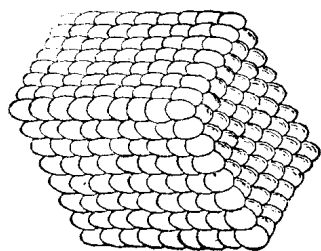
M. B. 羅蒙諾索夫 (1711—1765 圖 3. 方解石構造(按惠更司)
