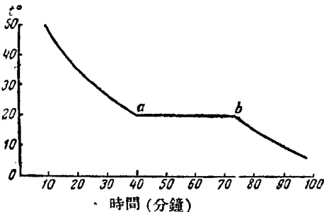
圖 7. 結晶物質的冷却曲線。
