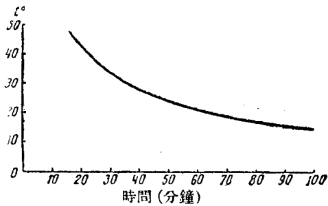
圖 6. 非晶質的冷却曲線。
