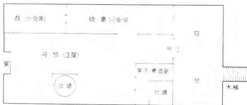
墨脱县门巴族住宅平面示意图
