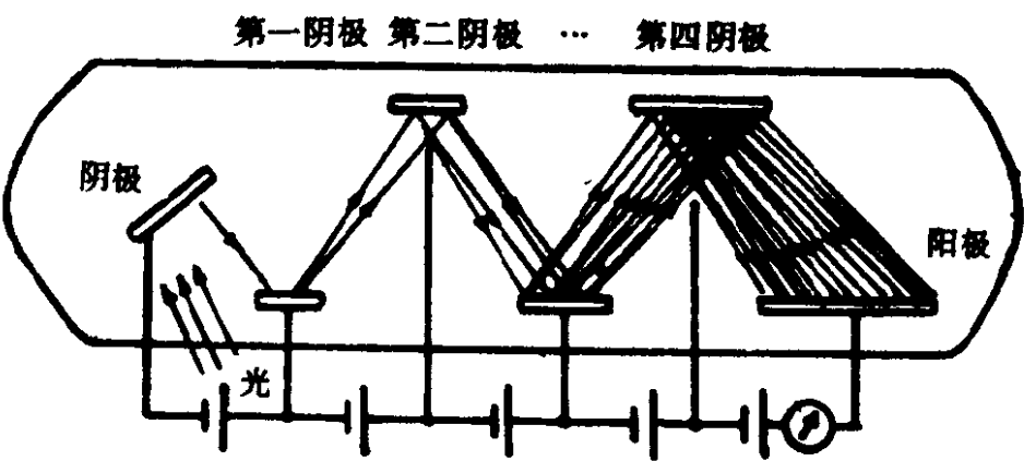
图 1-3 光电倍增管
