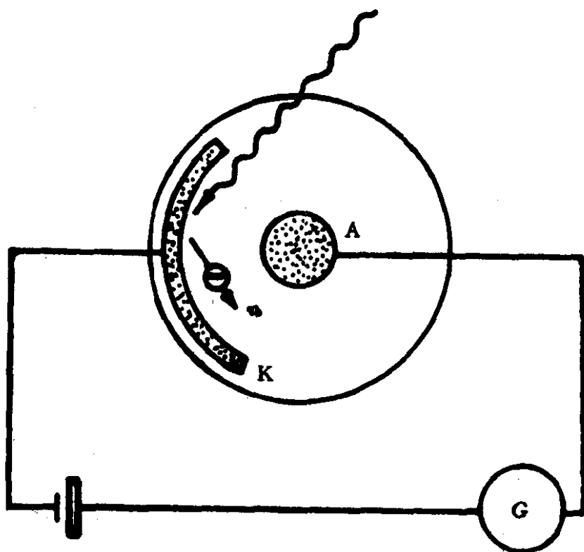
图1-1 外光电效应观察装置
