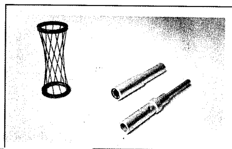
線簧結構
