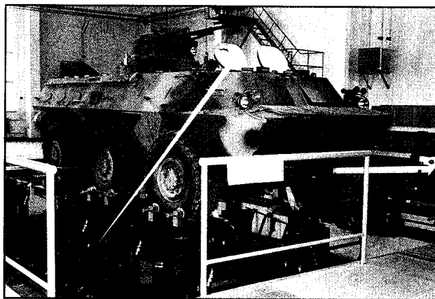
正在做战车试验的道路模拟试验台
