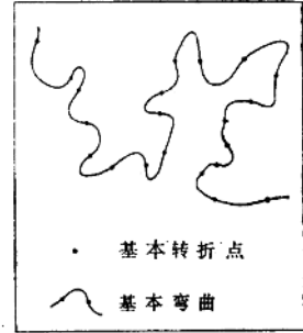
图 9-10 基本转折点和基本弯曲
