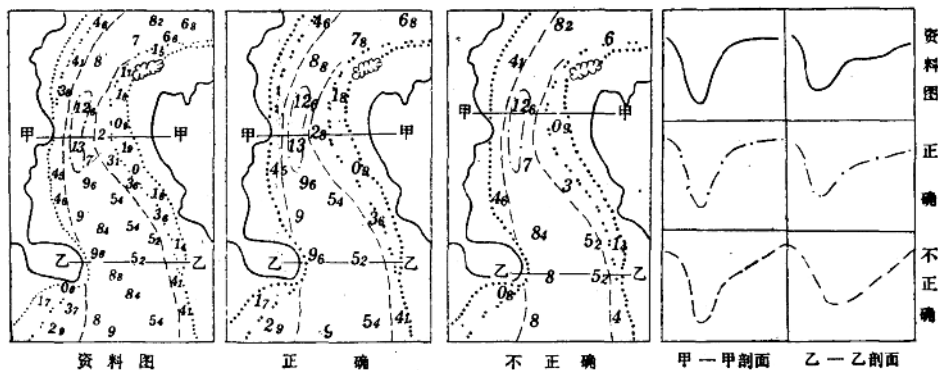
图 9-14 选取能反映航道宽度的水深
