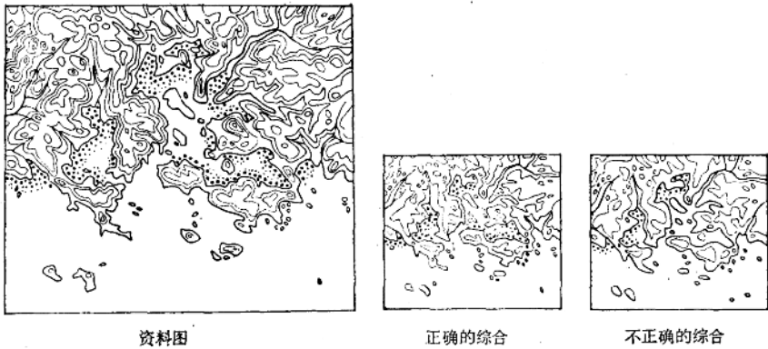
图 9-3 地形图上侵蚀海岸的概括示例
