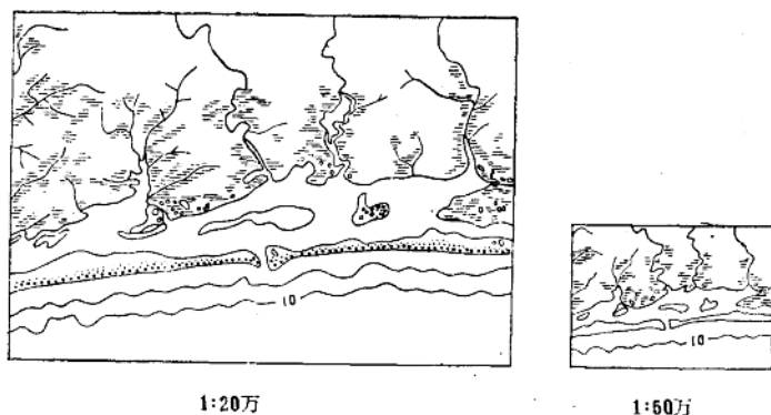
图 9-5 地形图上表示的泻湖型海岸
