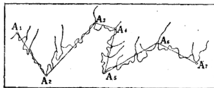
图 9-8 海岸线的曲线长和直线长
