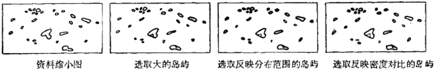
图 9-12 群岛中岛屿的选取步骤
