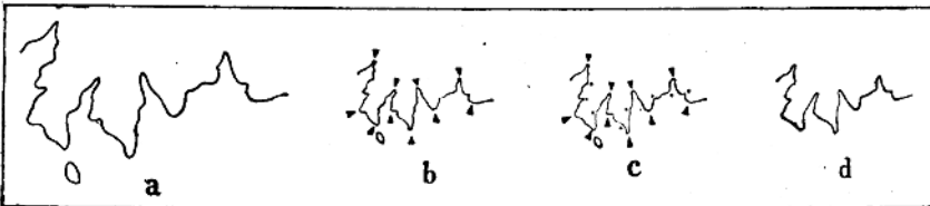
图 9-2 海岸线图形概括的方法和步骤
