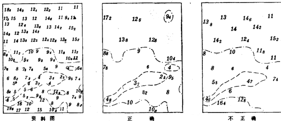
图 9-13 优先选取浅滩上最浅的水深
