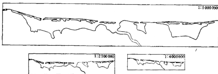
图 9-6 小比例尺地图上泻湖型堆积海岸的概括示例
