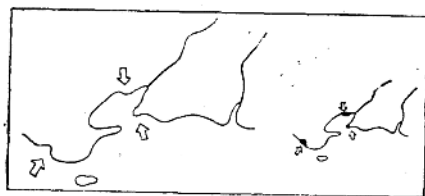
图 9-7 保持海陆面积对比的概括（放大图）
