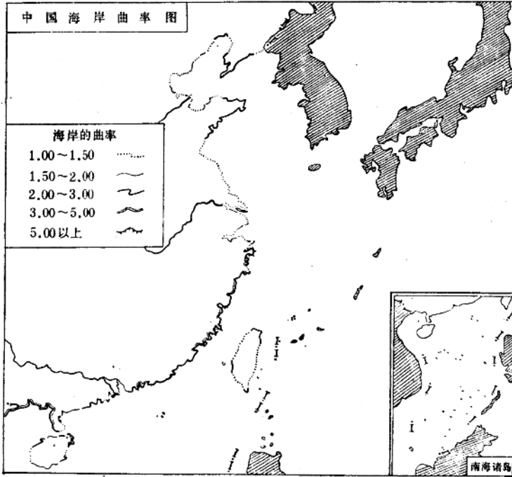
图 9-9 中国海岸曲率图
