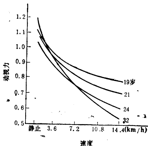
图 2-2 不同年龄时车速与动视力的关系
