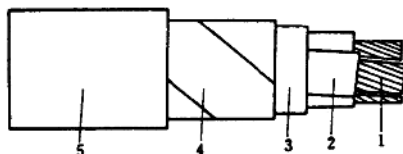
图 1-3 1 kV 聚氯乙烯绝缘内
