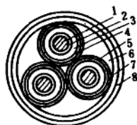
图 1-12 分相铅包电力 电缆结构图
