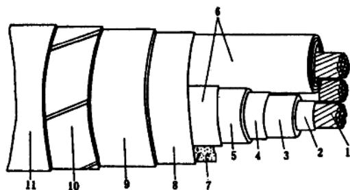
图 1-7 35 kV 三芯分相铅包油纸
