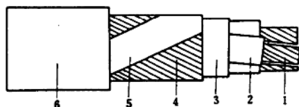
图 1-4 6 kV 聚氯乙烯绝缘三芯电缆
