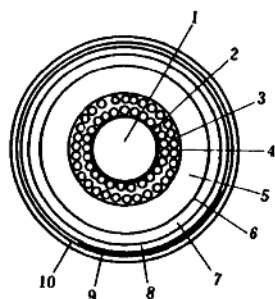
图 1-13 单芯自容式充油电力电缆结构图
