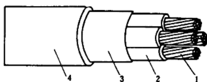
图 1-2 1 kV 聚氯乙烯绝缘四芯电缆
