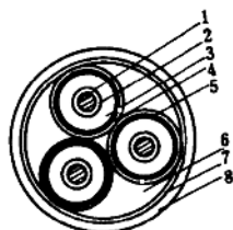
图 1-16 橡皮绝缘电力电缆结构图
