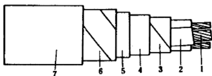
图 1-1 1 kV 油浸纸绝缘三芯电缆
