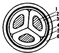
图 1-14 聚氯乙烯电力电缆结构图
