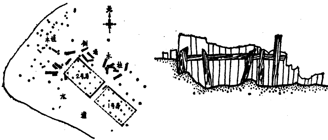
图 1-19 湖北圻春西周干阑建筑遗址 (左图—水塘中木架建筑遗存; 右图—一部分木外墙遗物)
