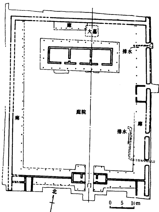
图 1-14 河南偃师二里头二号宫殿遗址平面
