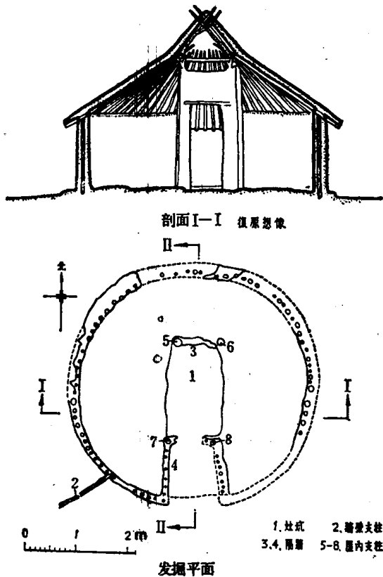
图 1-5 西安半坡 F 41 半穴居建筑遗址平面
