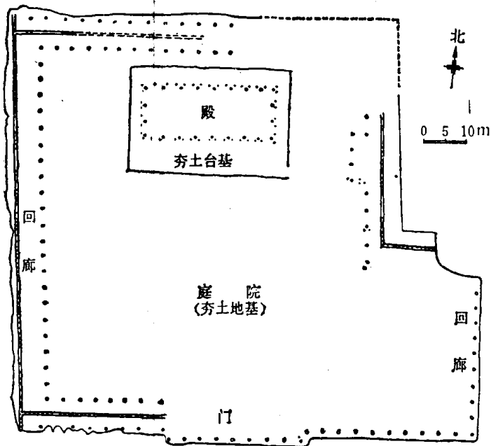
图 1-13 河南偃师二里头一号宫殿遗址
