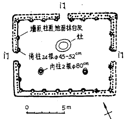
图 1-6 甘肃秦安大地湾 F 405 仰韶晚期房屋遗址平面
