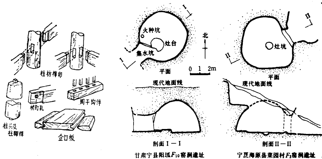
图 1-2 原始社会窑洞住宅遗址二例
