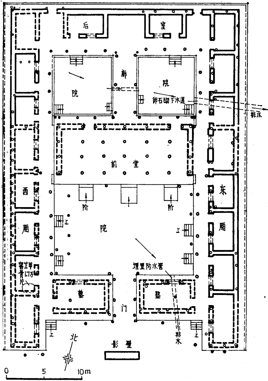
图 1-18 陕西岐山凤雏村西周建筑遗址平面
