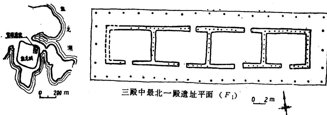
图 1-15 湖北黄陂县盘龙城商代宫殿遗址
