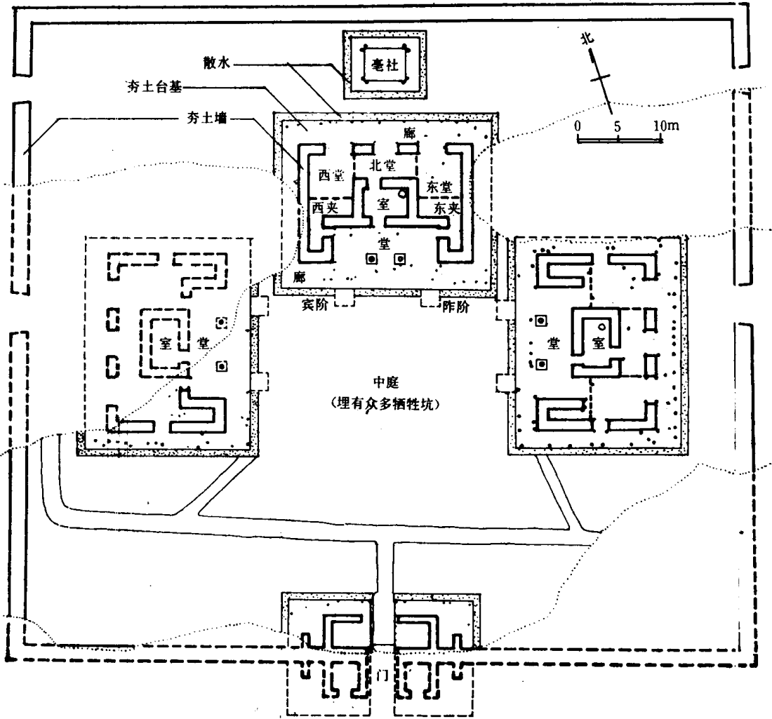
图 1-22 春秋时期秦国宗庙遗址平面（陕西凤翔马家庄一号建筑遗址）
