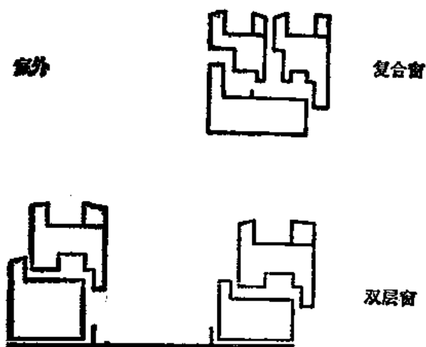
图 2—4 多扇系列的垂直剖面
