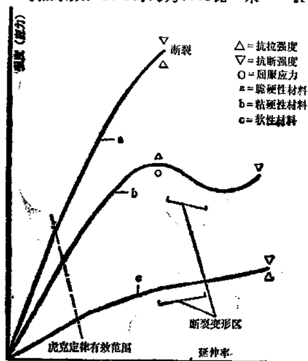
图1-1 各种热塑性塑料的应力应变图
