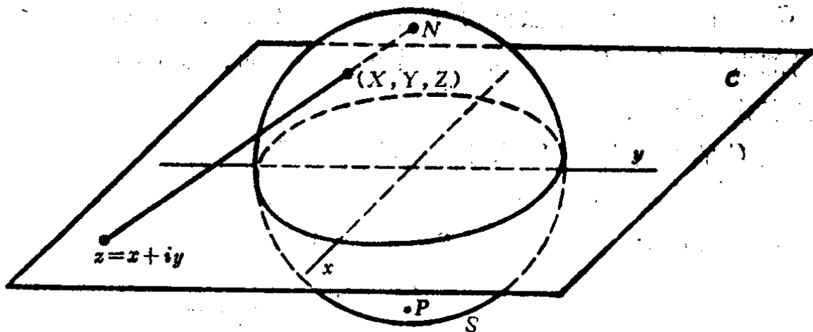
图1.1 球极投影
