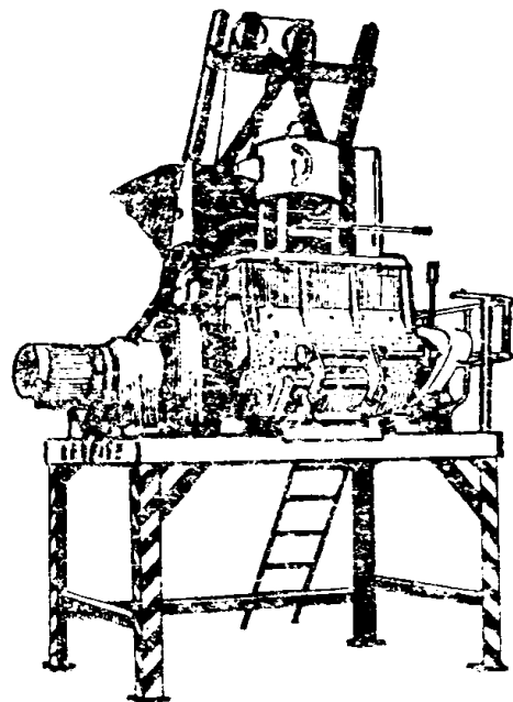
建设部1987年度优质产品 JS350型双卧轴强制式搅拌机 (出料容量350L)
