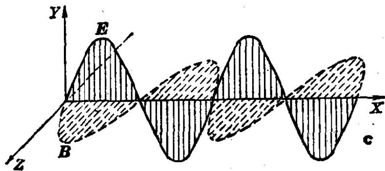
图 1-1 电磁波
