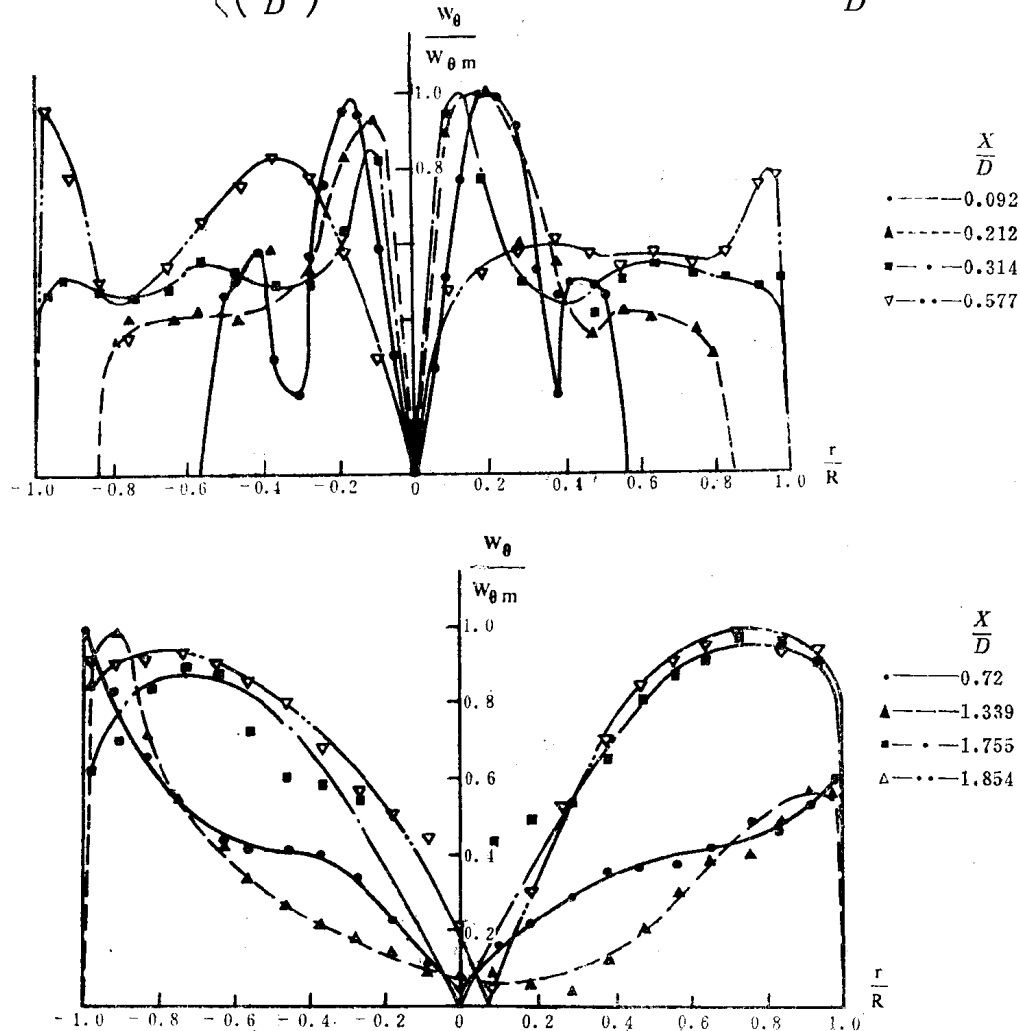
图9 切向速度的径向分布图
