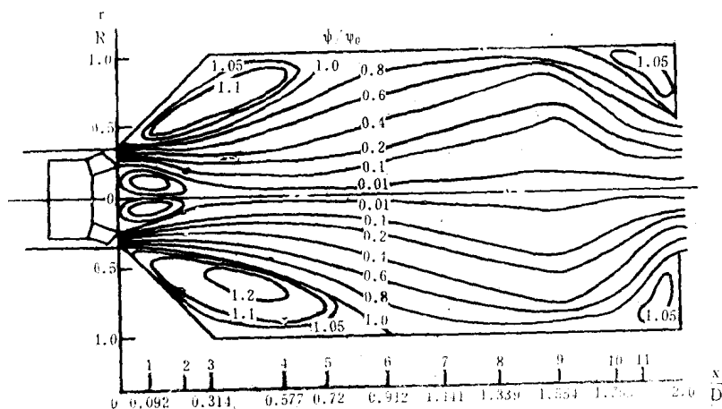
图 5 燃烧室中气流流线图 ( w_D = 11.75 米/秒)
