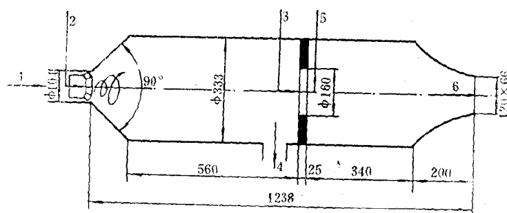
图 1 JS-2燃煤MHD燃烧室示意图
