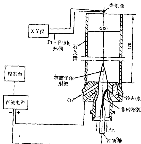
图1 试验系统图
