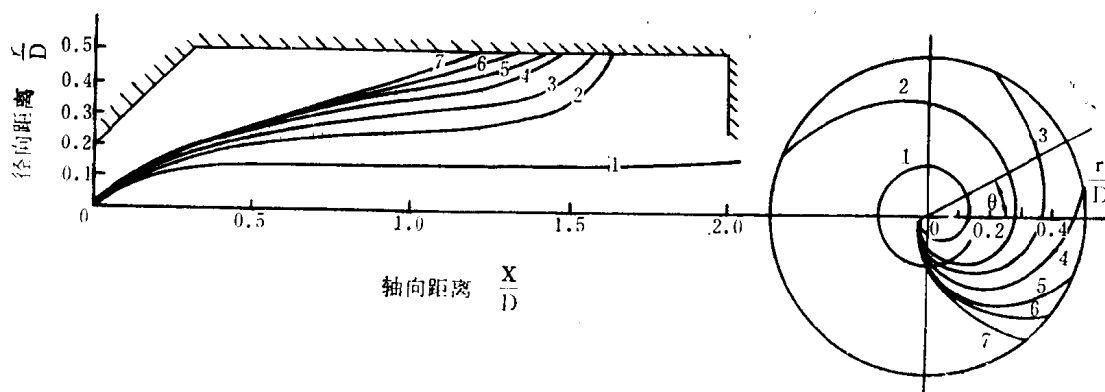
图 10 煤粉颗粒在燃烧室中的运动轨迹
