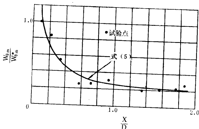
图7 最大切向速度沿轴线的衰减情况
