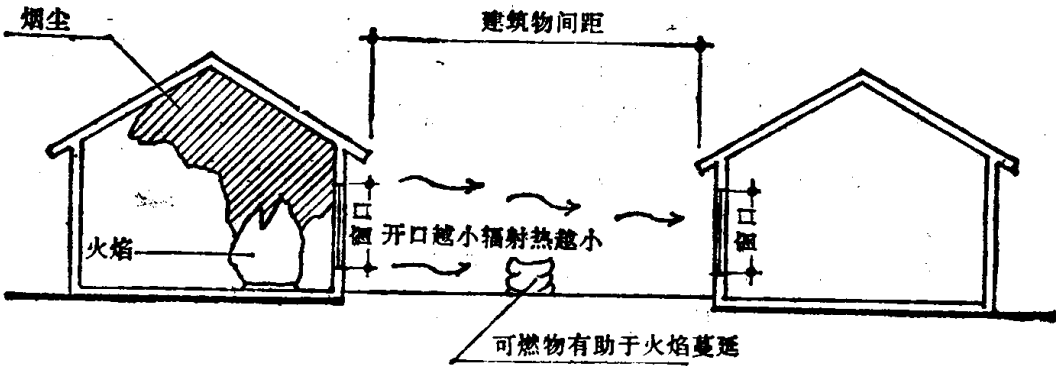
图 1-3 建筑物的辐射途径
