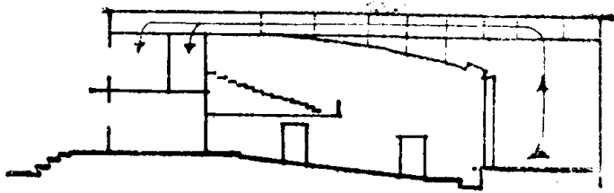
图 1-1 剧场火势蔓延途径 △一起火点： →—火势蔓延途径
