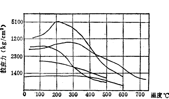
图 1-5 金属强度随温升的变化
