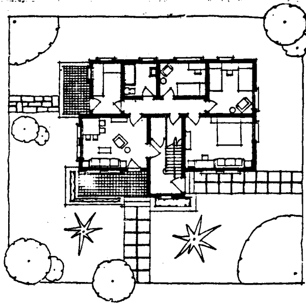
一层平面
