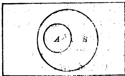
图1-1 B \supset A
