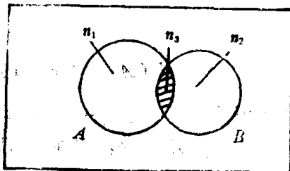
图1-6 A 、 B 发生情况
