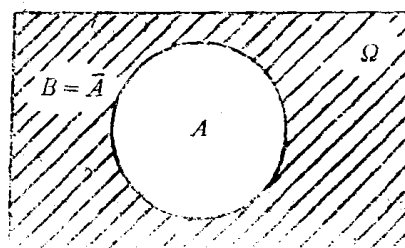
图1-4 A 与 B 互逆
