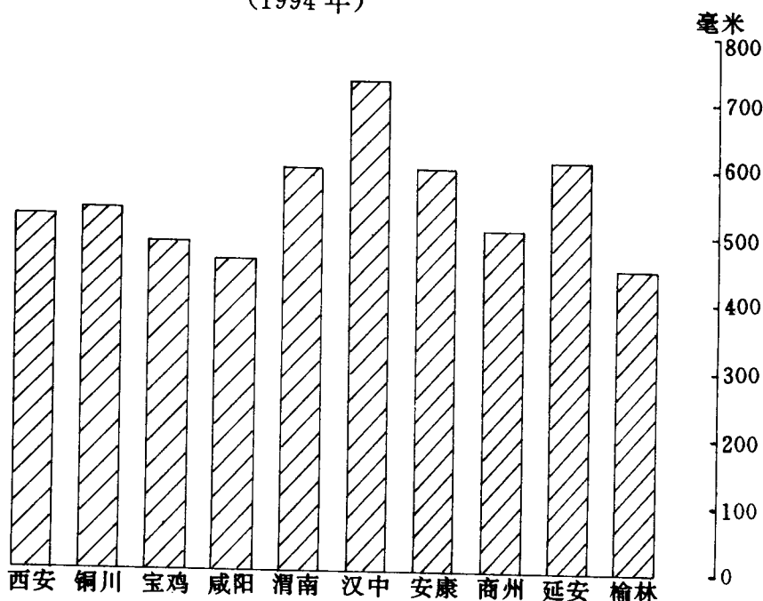
主要城市降水量 (1994 年)
