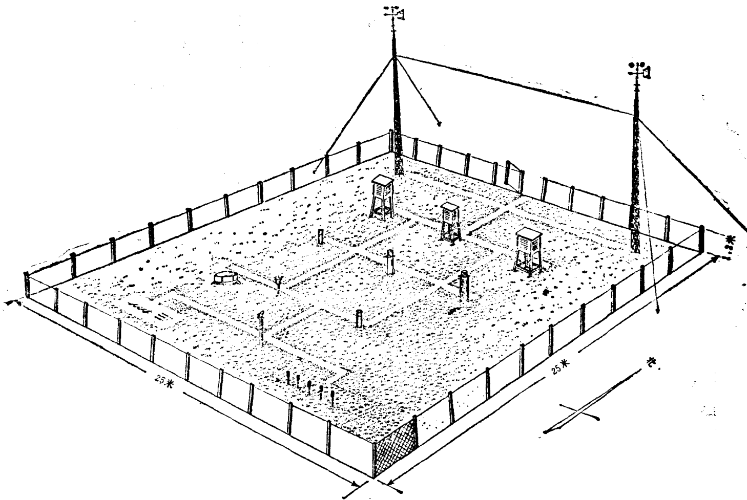
图 1.1 观测场仪器布置参考图
