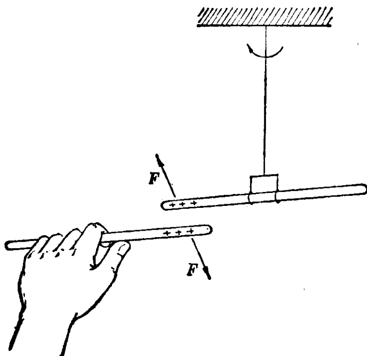
图 1-1 带电玻璃棒之间的相互排斥
