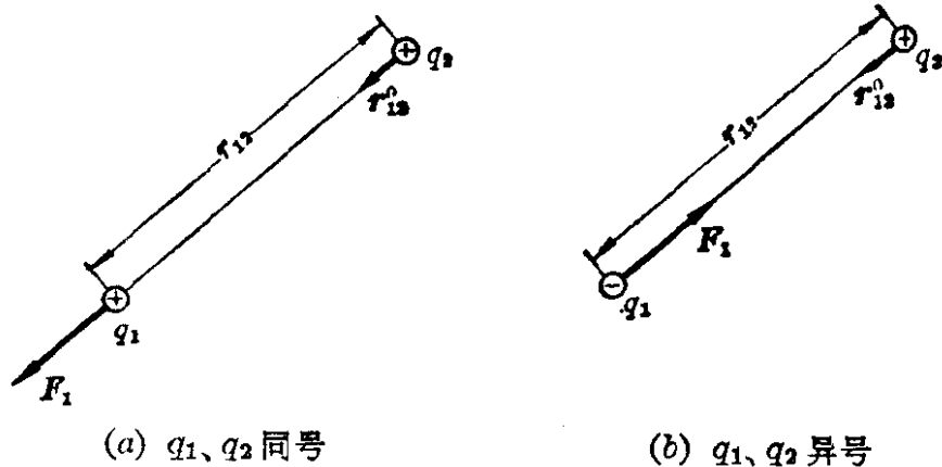
图 1-2 点电荷 q_2 对 q_1 的作用力
