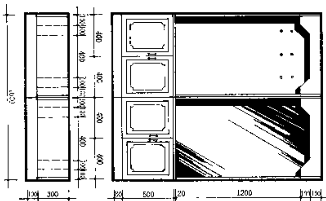
图 11-1 窗面家具之
