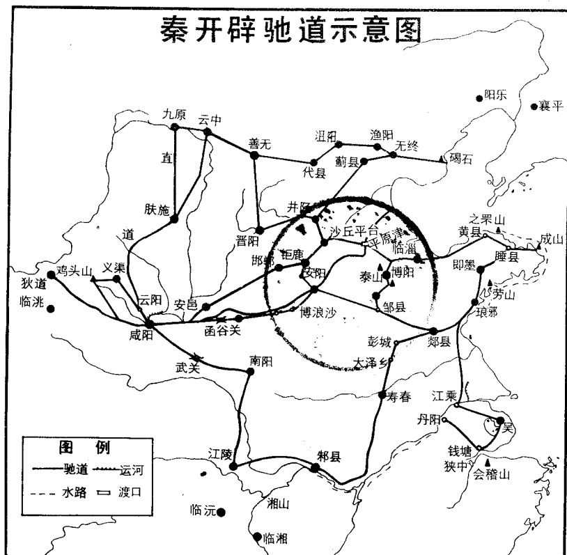
秦代驰道图
