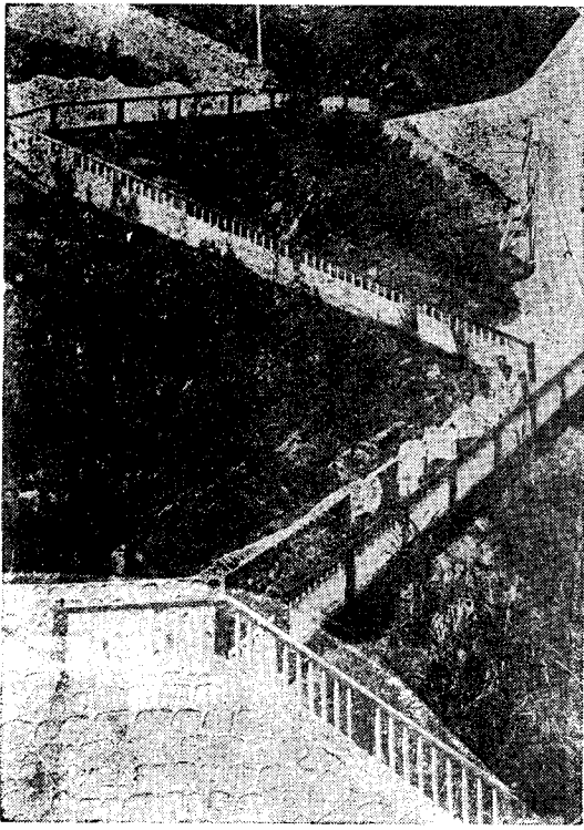
坐落在瑶区的三水电站拦河大坝一角
