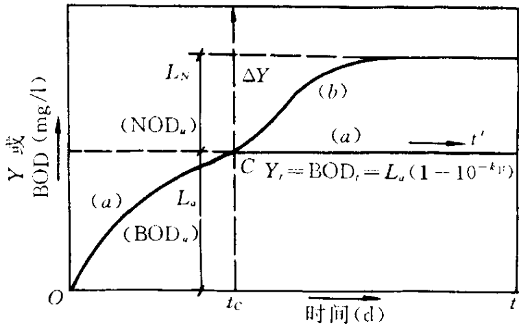
图 2-2 BOD 曲线
