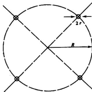
图 A3 等效半径计算图
