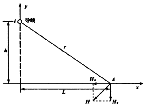
图 B1 磁场向量图
