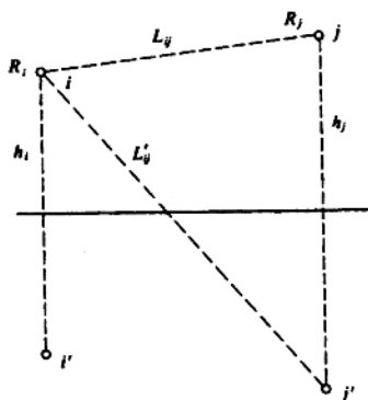
图 A2 电位系数计算图
