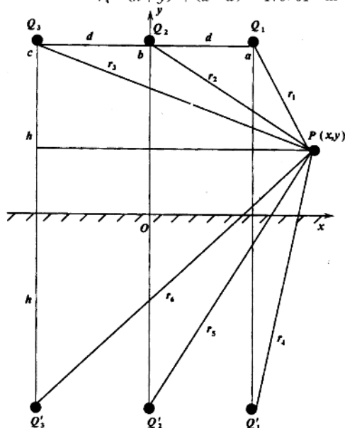
图 A5 各导线坐标图
