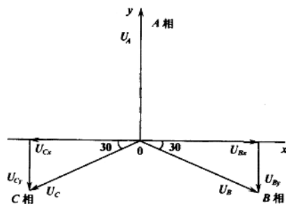
图 A1 对地电压计算图
