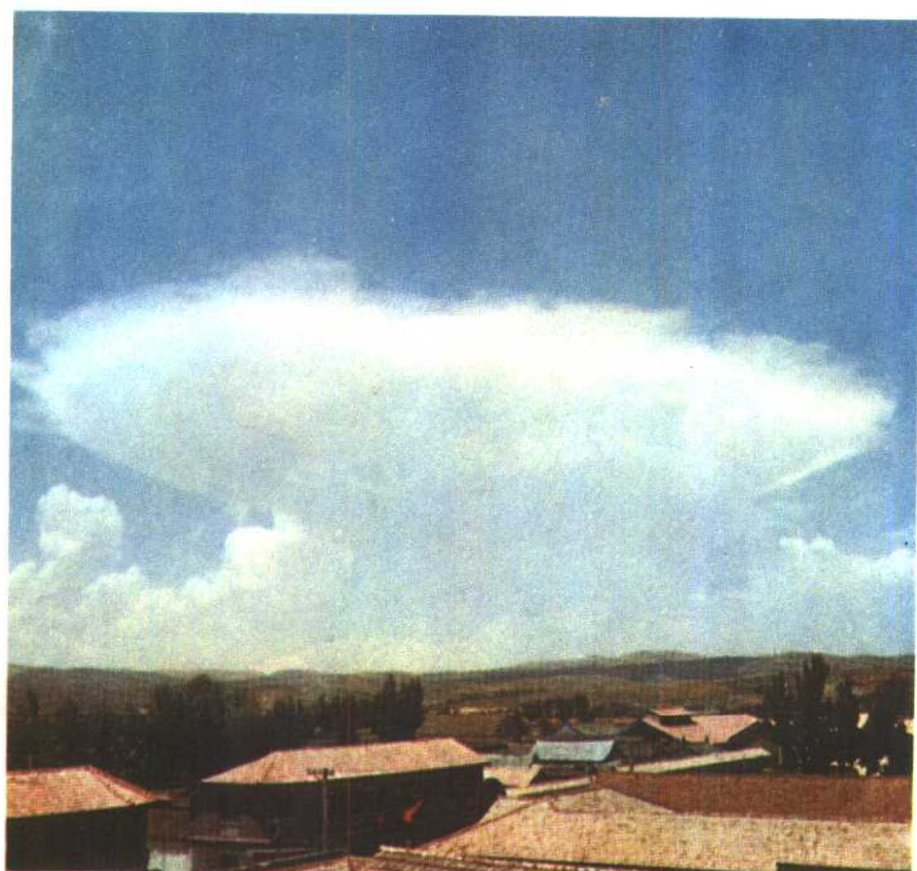
图 2 | 21 砧积雨云
