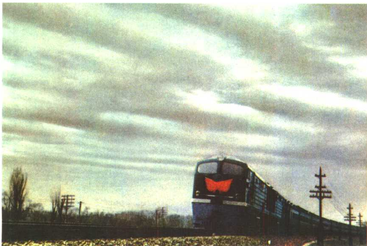
图2-23 透光层积云
