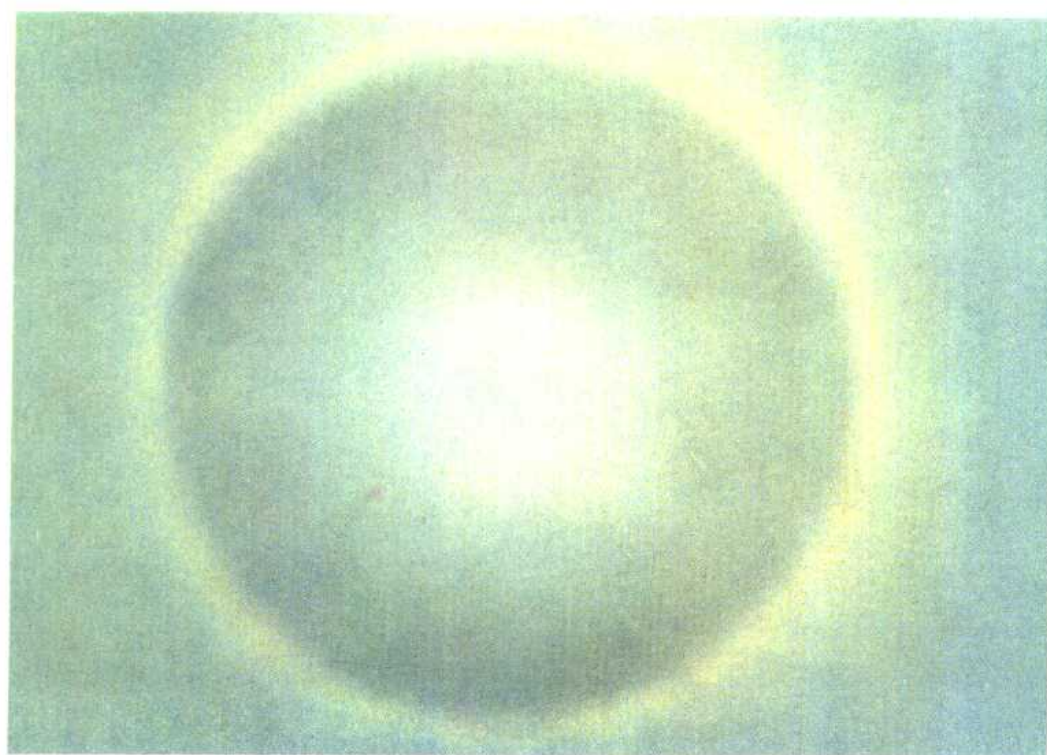
图 2 | 46 毛卷层云
