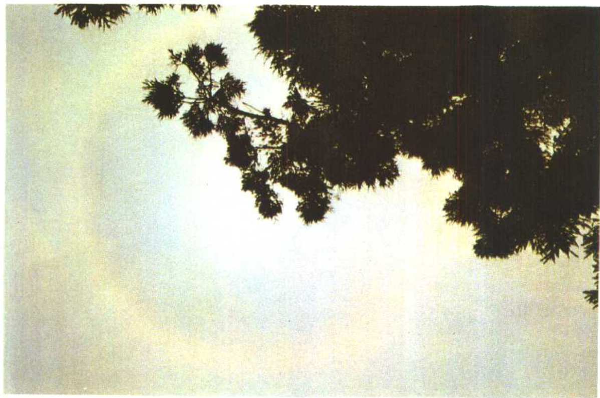
图2-45 匀卷层云
