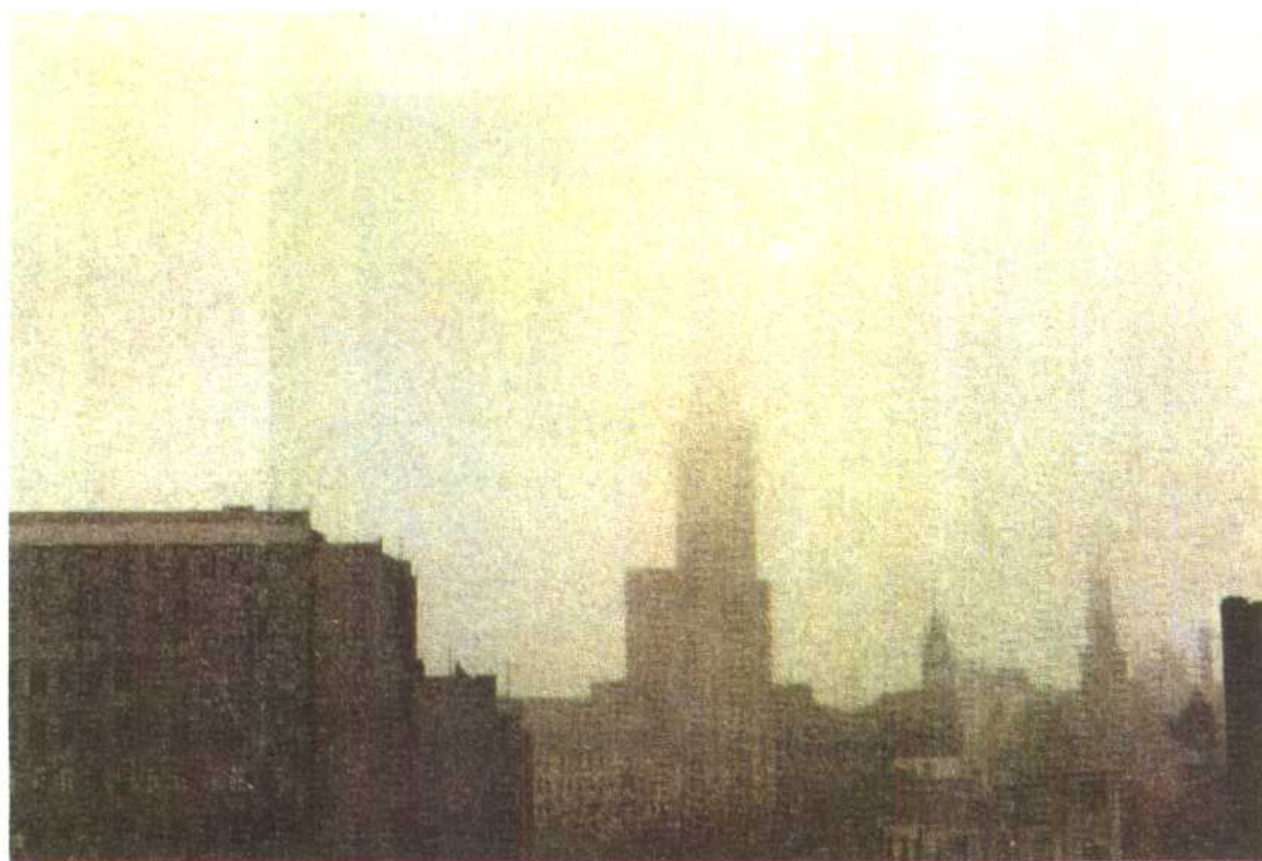
图2-27 层 云
