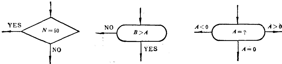
图 2-4 判断框的三种表示
