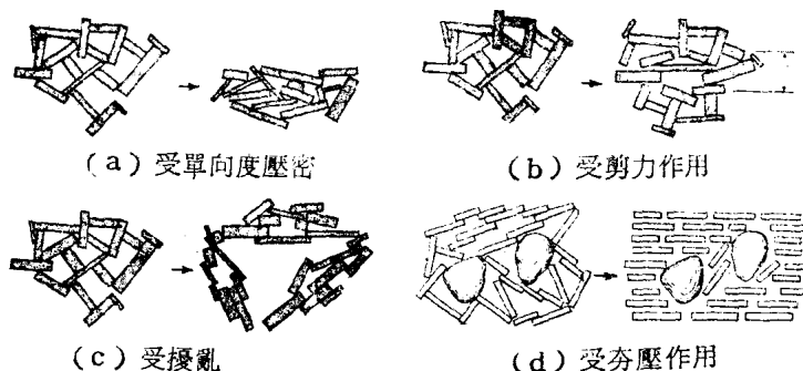
圖 1.6 飛架結構受擾動後顆粒排列的變化
