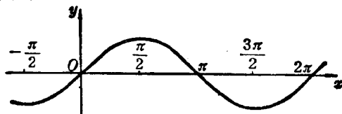
图 1-1 y = \sin x
