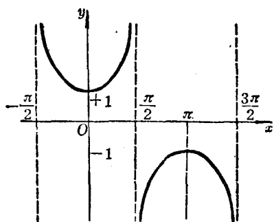
图 1-4 y = \sec x
