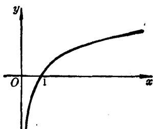
图 1-6 y = \lg x
