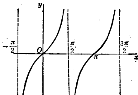
图 1-3 y = \text{tg } x
