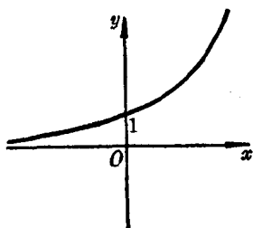
图 1-5 y = a^x (a > 1)
