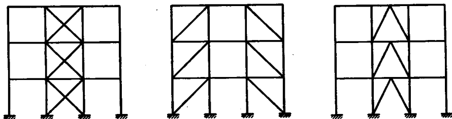
图 1-2 各种中心支撑框架结构
