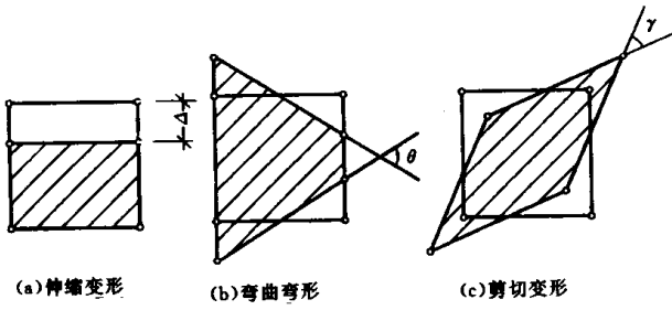
图 1-8 节点域的变形
