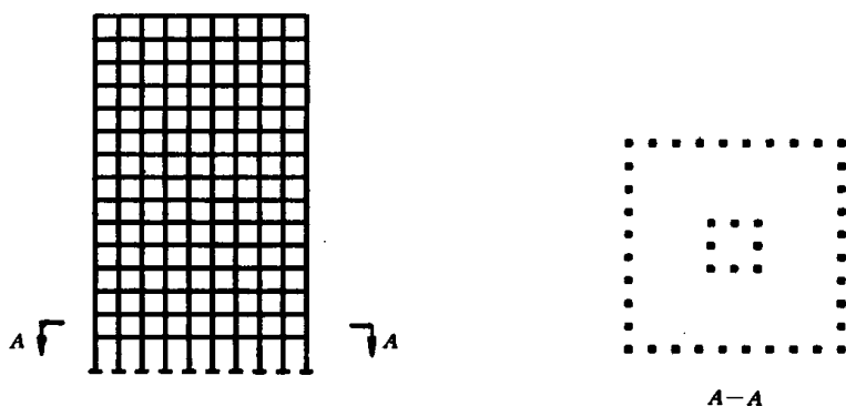
图 1-4 框筒结构
