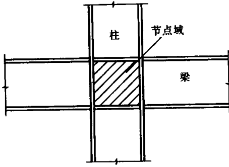
图 1-7 钢框架节点域
