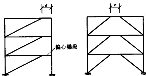
图 1-3 偏心支撑框架结构
