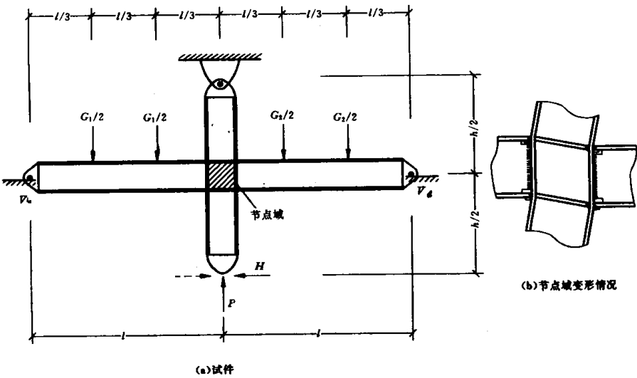
图 1-9 钢框架节点域试验
