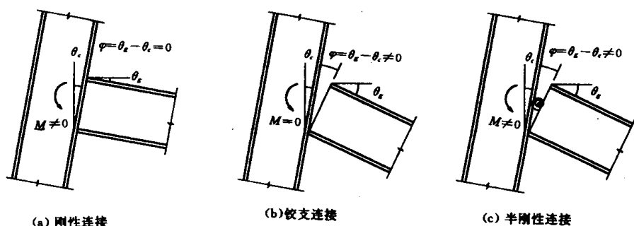
图 1-5 钢框架梁柱连接的受力与变形
