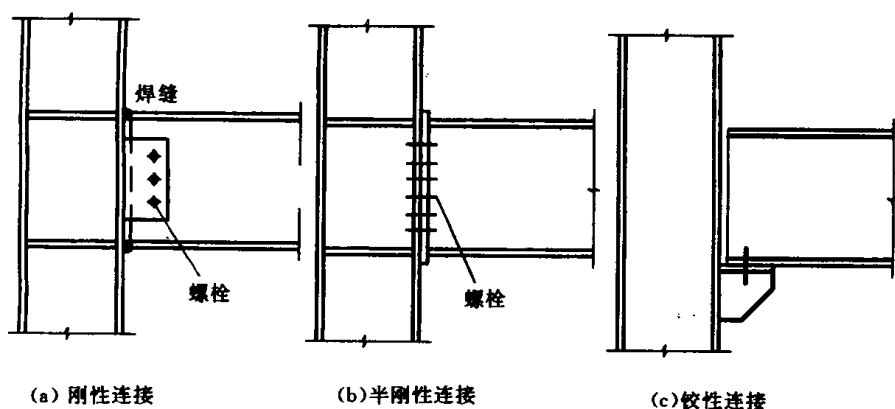
图 1-6 钢框架梁柱连接的典型构造形式
