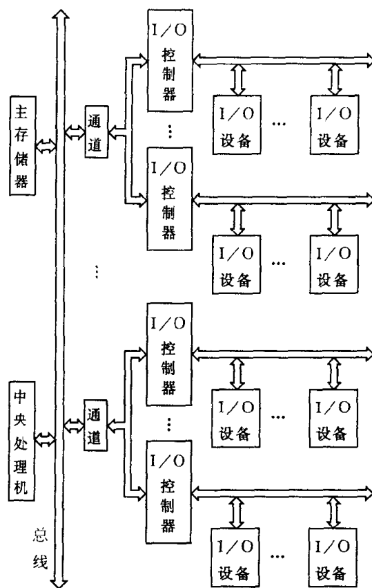
图 1.4 大、中型计算机系统的通道型结构
