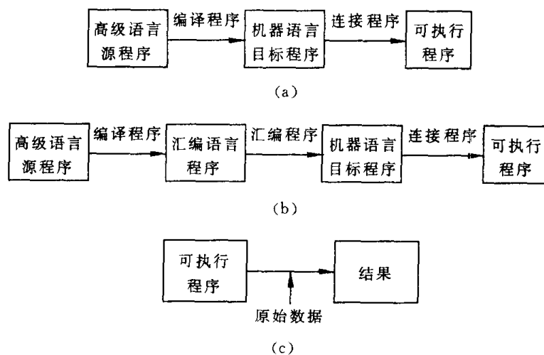
图 1.5 编译程序作用下源程序的执行过程
