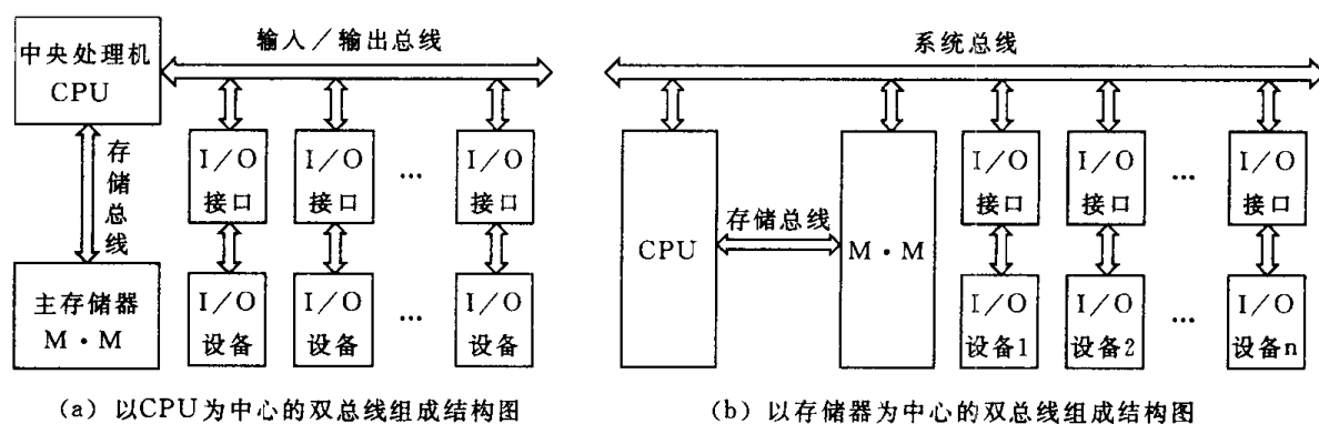
图 1.3 双总线结构
