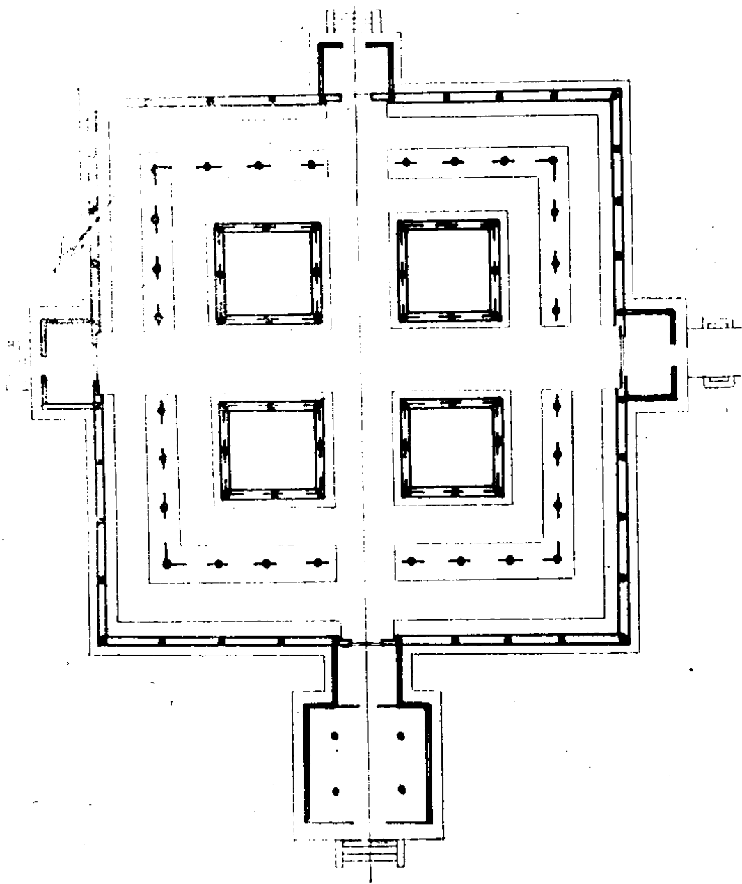
图1 罗汉堂平面图 北→
